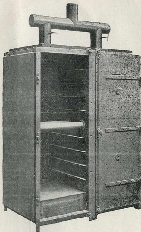
Etuve électrique double pour la cuisson des vernis, munie d'autorégulateur de température et réalisant une parfaite isothermie
